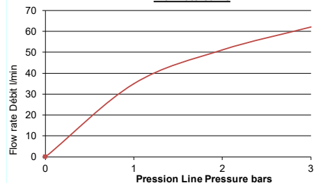
Courbe de débit Flow rate curve
